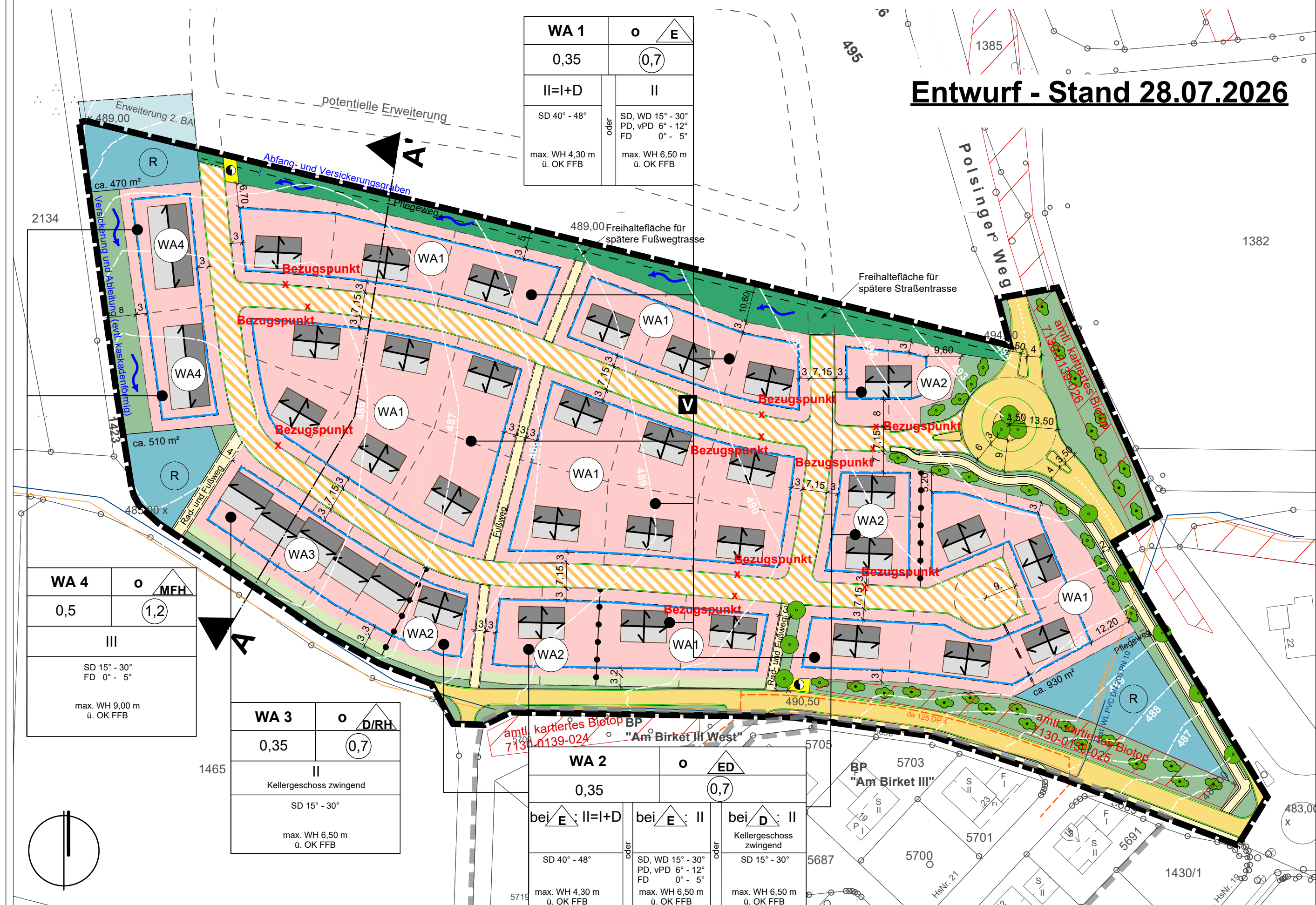
Teil A - Planzeichnung M 1:1.000
